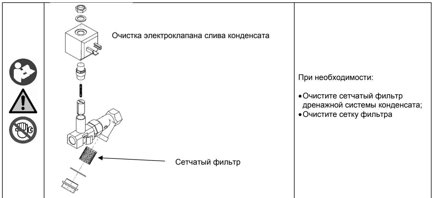
Рис. 3 электроклапана слива конденсата
